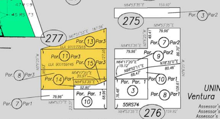
DETAIL 1 - LLA 000106191
